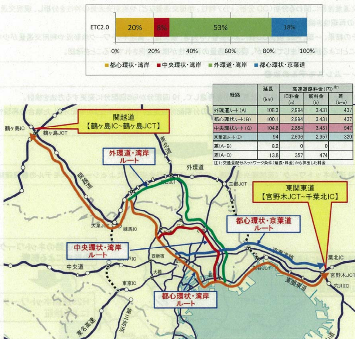
図 4-40 外環道・都心環状ルートの交通分担
