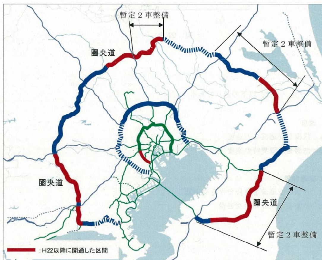
図 4-13 H28 高速道路ネットワーク（3環状関連）
