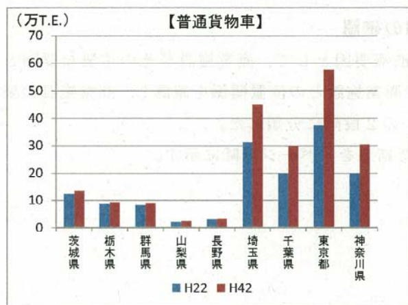
図 6-13 発生集中交通量（都県内外交通）
