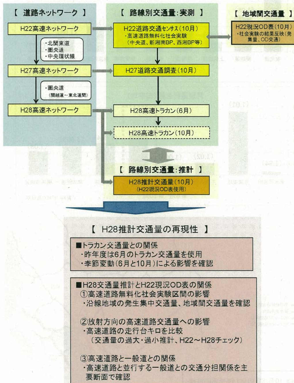
図 4-2 再現性検証フロー
