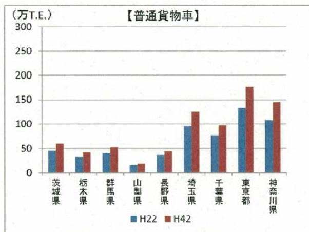
図 6-14 発生集中交通量（都県内々交通）
