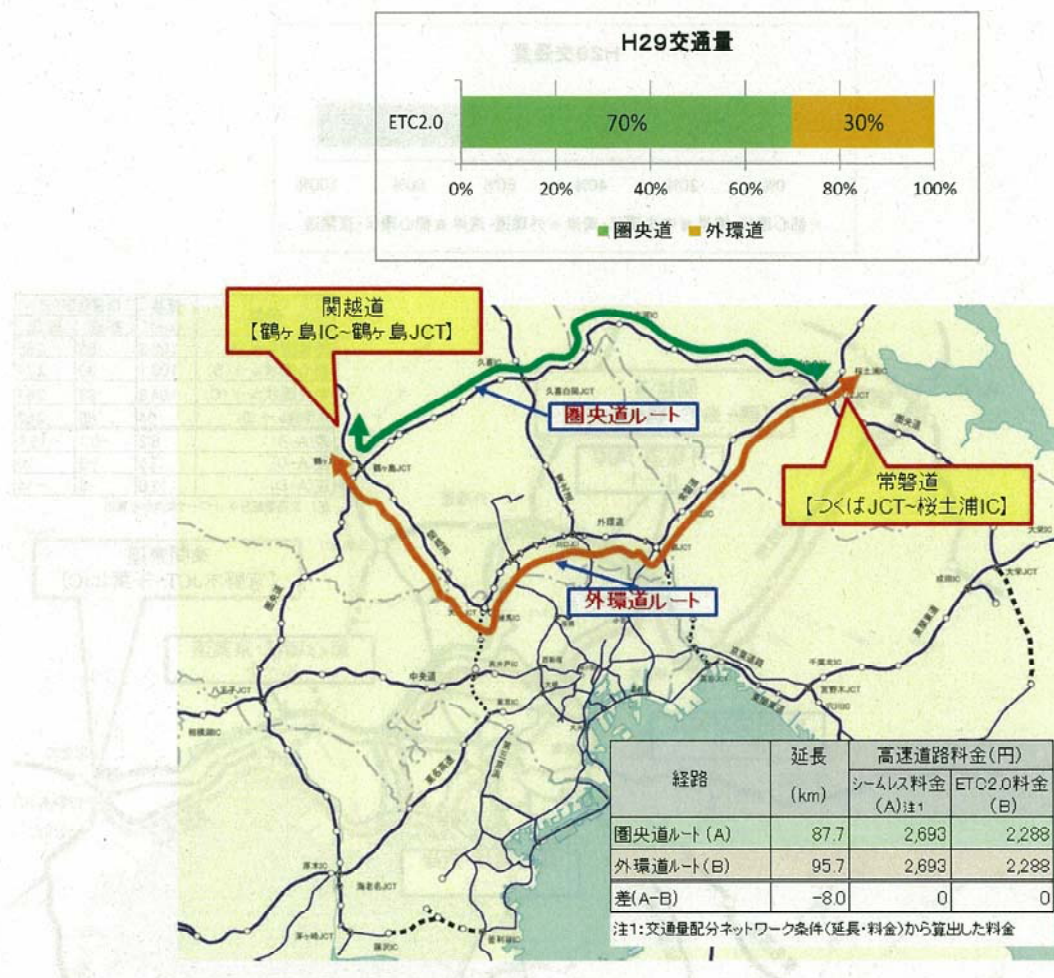
図 5-15 圏央道・外環道ルートの交通分担
