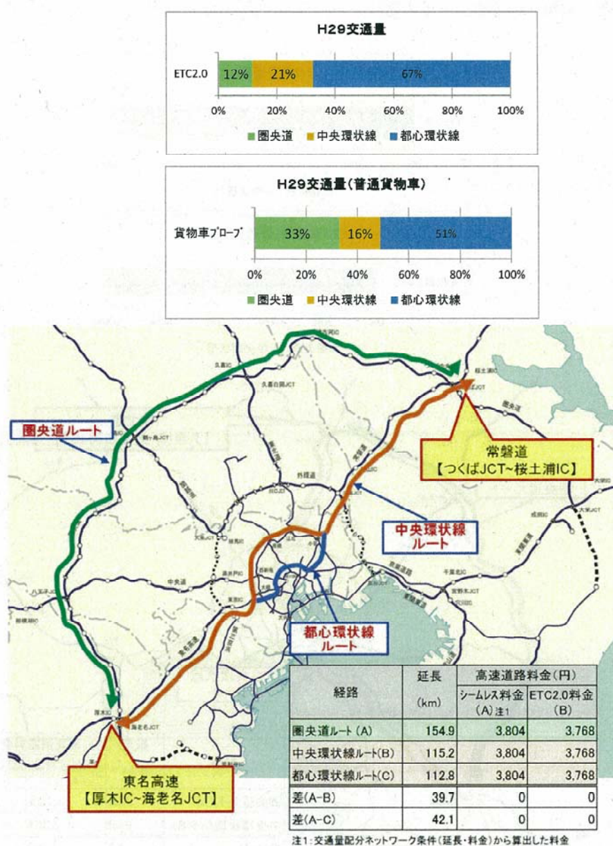
図 5-10 圏央道・中央環状線・都心環状線ルートの交通分担
