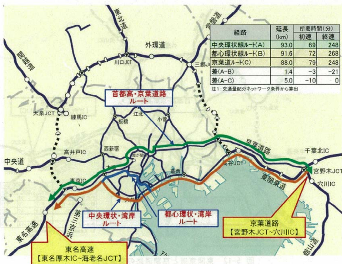
図 5-11 東関東道と京葉道路の交通分担
