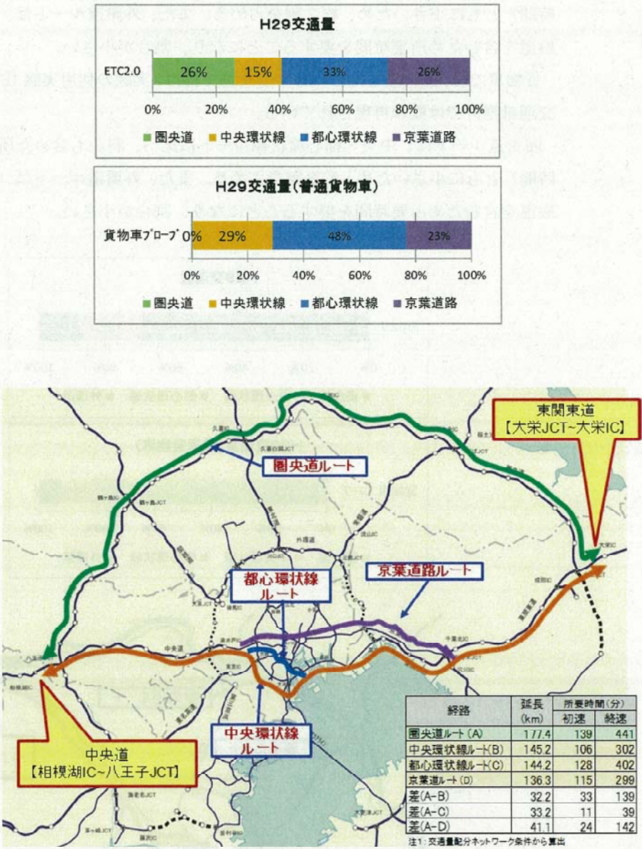
図 5-14 圏央道・中央環状線・都心環状線・京葉道路ルートの交通分担
